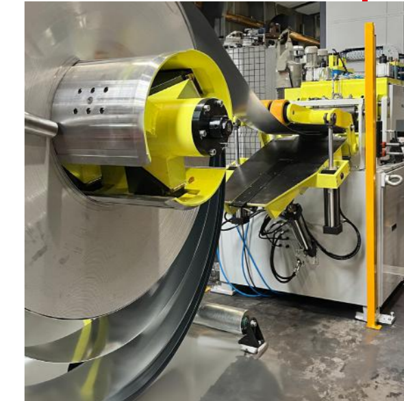
Haspel mit Schnellrüster Millutensil Richtapparat
